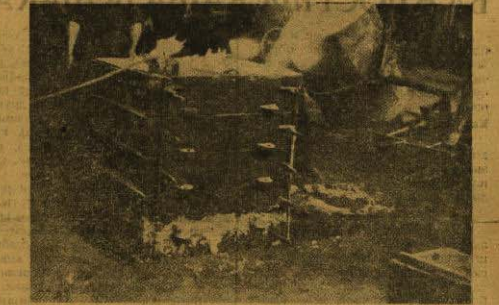
У ОВОМ ВЕЛИКОМ КАЛУПУ ИЗРАДИЋЕ СЕ ОСОВИНА ЗА ПЕЋ, КОЈА ЋЕ ПОСЛУЖИТИ ЗА ЛИВАЊЕ ЂЕЛИКА, ОСОВИНА ЋЕ БИТИ ТЕШКА ОКО 500 КГ.
