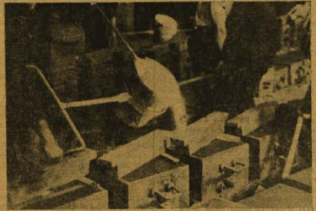
У КАЛУПЕ СЕ ЛИЈЕВА УСИЛАНО, ТЕКУЋЕ ЖЕЛЕЗО. КАД СЕ ОНО ОХЛАДИ ДОБИЉЕМО СЈЕКРЕ, НАКОВЊЕ, ДИЈЕЛОВЕ СТРОЈЕВА И ДРУГО
