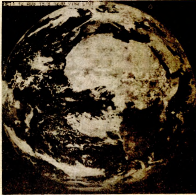
Geostacionarna orbita: Zemlja videna sa 36 hiljada kilometara
