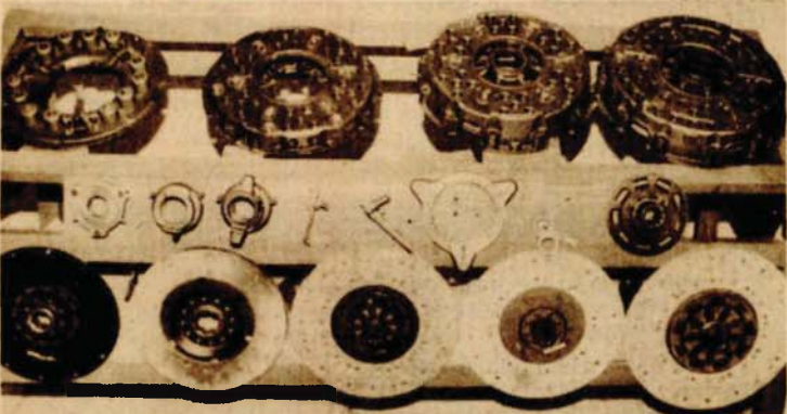
Dijelovi spojnice iz osnovnog programa FAMOS—ove Fabrike u Sanskom Mostu
