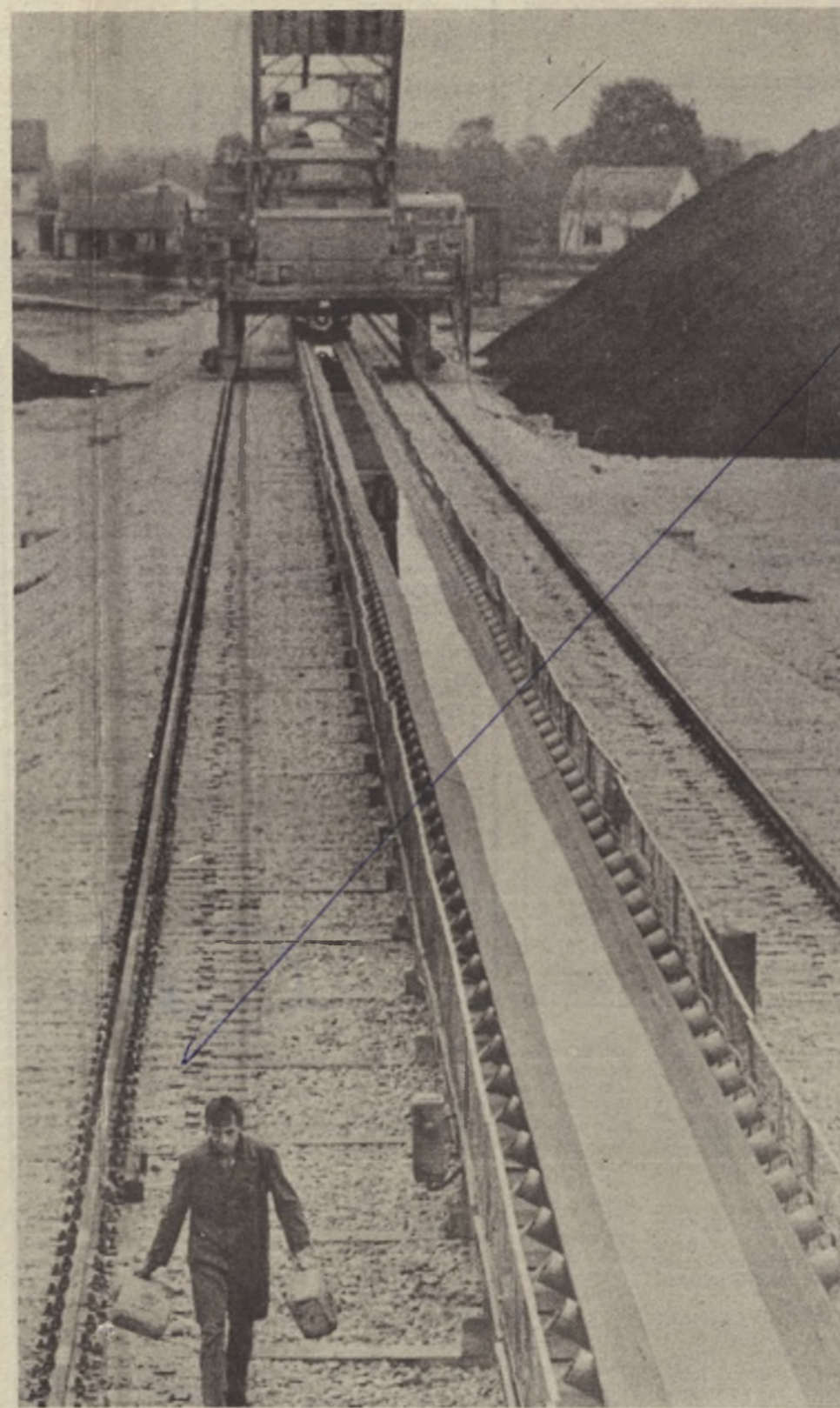
Željezna ruda automatskim putem stiže do elektromagnetne separacije, gdje se vrlo fino odvajanje od ostatka jalovine. U neposrednoj blizini moćnih transportera magnetne filtracije nalazi se željeznička stanica, sa manevarskim prostorom, dovoljnim da ruda na najbrži način bude odvožena do željezara
