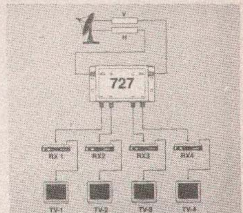
Шема прикључења четири корисника на једну сателитску антену
