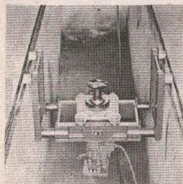
HIDROPNEUMATSKA KANALNA DIZALICA NOSIVOST 80-150 kN
