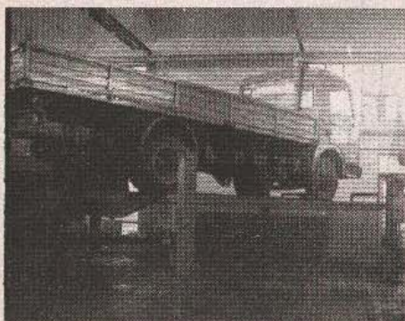
ELEKTROMEHANIČKA ČETVEROSTUBNA DIZALICA DF1, NOSIVOST 50 kN
