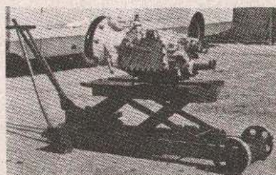
HIDRAULIČNA KOLICA CM3 NOSIVOST 22 kN
