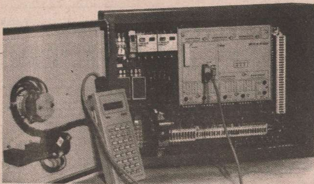
Комплетно ел. управљање за хидрауличке универзалне маказе, остварено програмабилним аутоматом.
