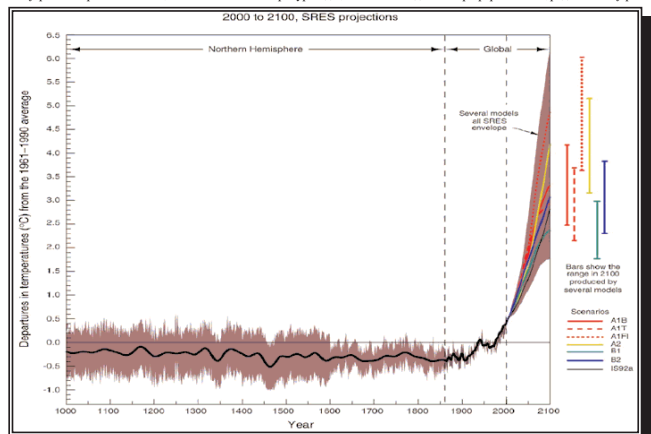
Пројекције раста средње глобалне температуре ваздуха у 21. вијеку (Извор: ИПЦЦ, 2001)
