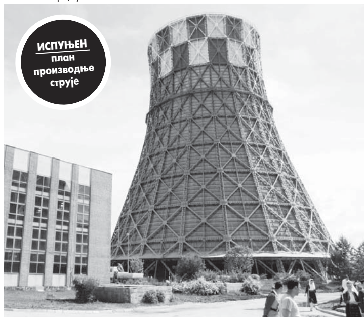
Термоелектрана "Гацко"
