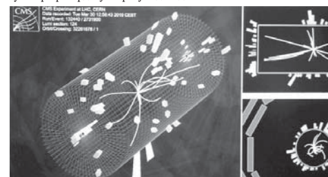
Судар субатомских честица
