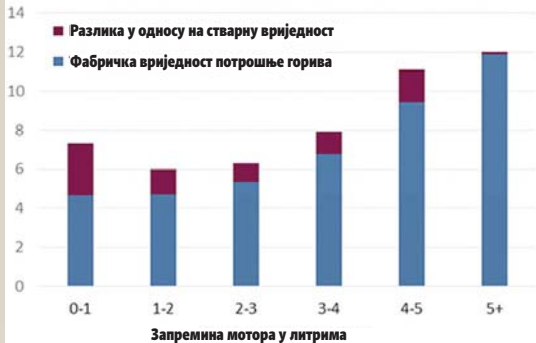
Измјерена потрошња горива у l/100 km
