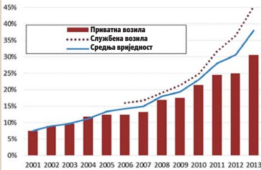
Стварна потрошња горива - прекорачење фабричких вриједности у постоцима
