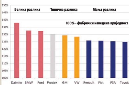
Стварна потрошња горива - прекорачење фабричких вриједности у постоцима
