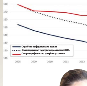
Просјечна емисија CO 2 нових аутомобила у г/км
